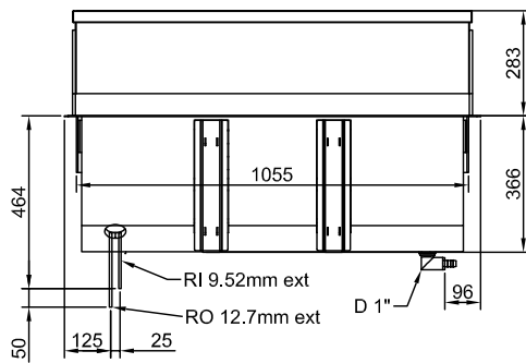
Lato posteriore
